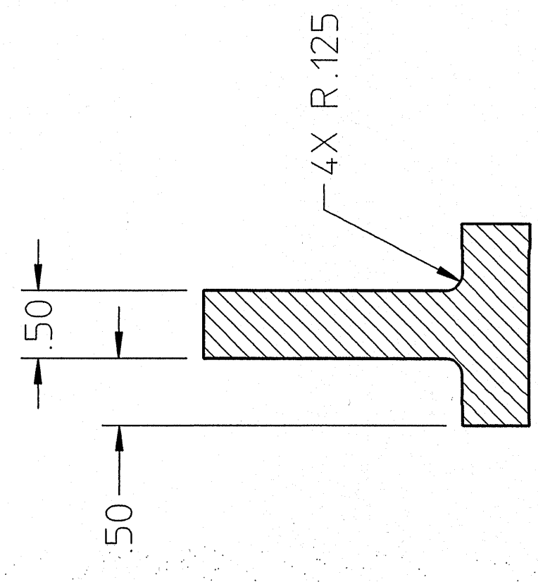
SECTION A-A
