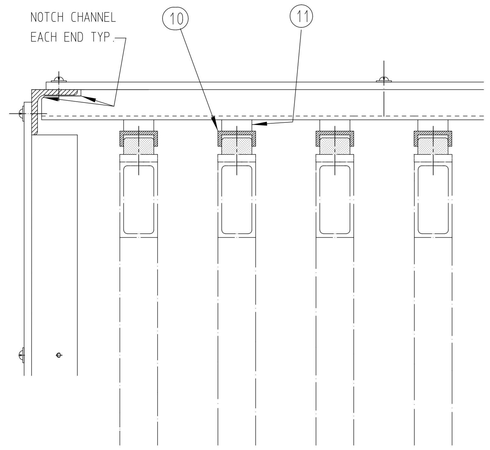
DETAIL "A" SCALE: HALF SIZE
